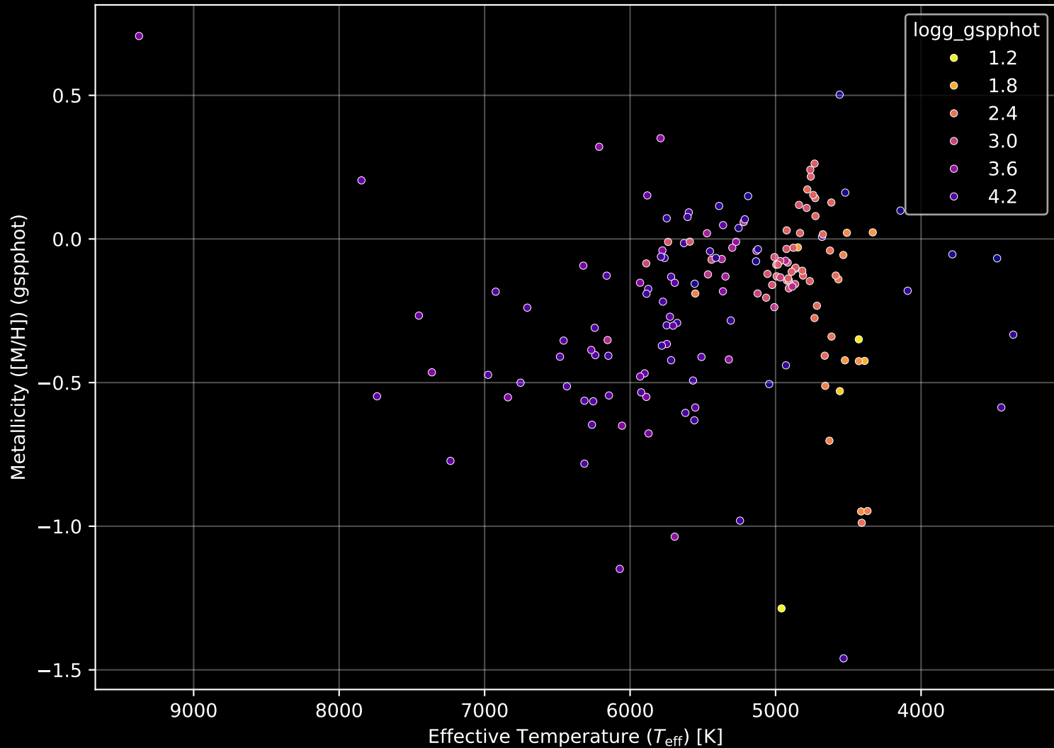
APOGEE DR17 Field: [272-22-O_TESS] Stellar Population Parameters (n= 163)
